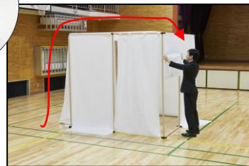
・天井(2枚)を被せる。
