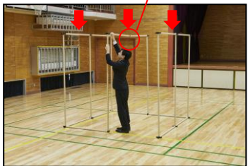
・天井フレーム(前後方向)を接続する
